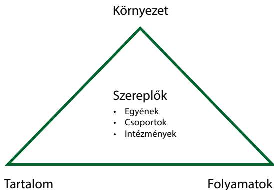
1. ábra: A szakpolitika elemzési kerete Walt és Gilson (1994) alapján
